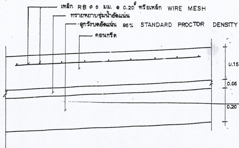
รายละเอียดคอนกรีตเสริมเหล็ก not to scale
