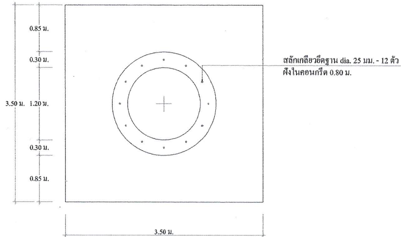
แบบขยายฐานรากหอดึงสูง (แบบฐานแม่) มาตราส่วน 1 : 50
