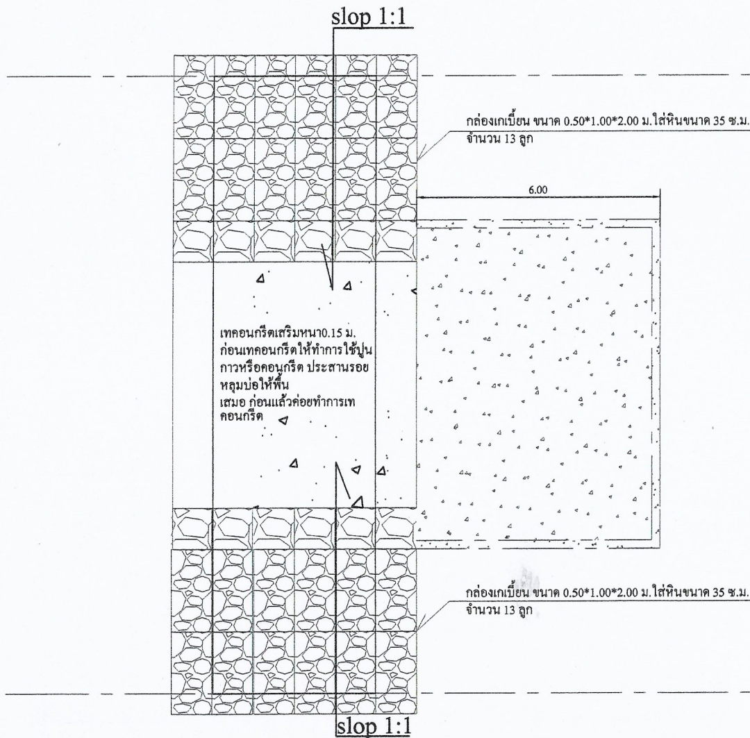
แปลนวางกล่องเกเบี้ยนชั้นที่ 2 NO SACL
