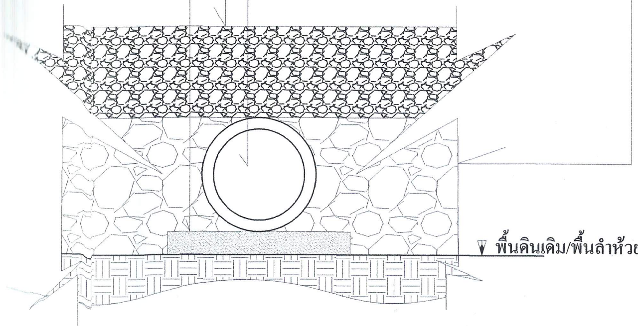
รูปตัดวางท่อระบายน้ำ NO SCALE
