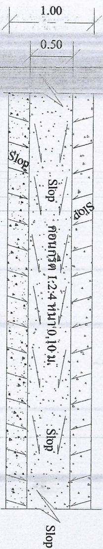
รูปรางระบายน้ำ NO SCALE
