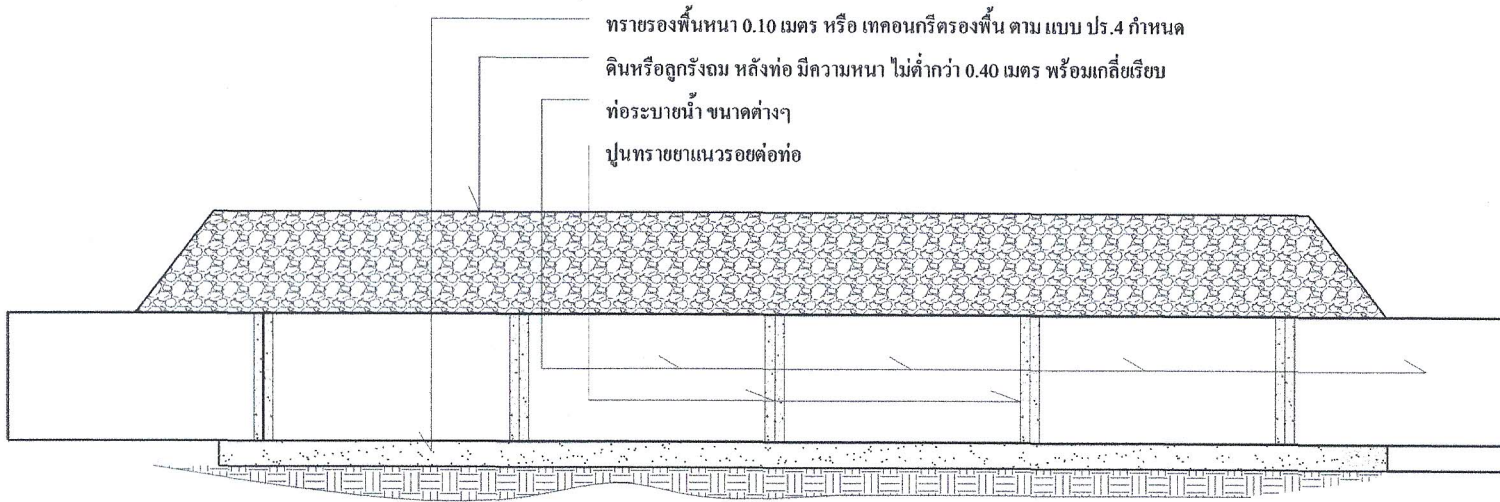
รูปตัดขวางท่อระบายน้ำ NO SCALE
