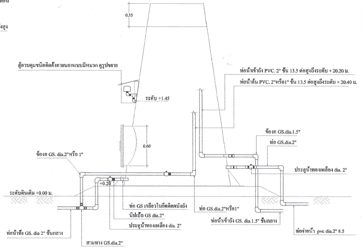
แบบแสดงการเดินท่อในถังแชมเปอู มาตราส่วน 1 : 25
