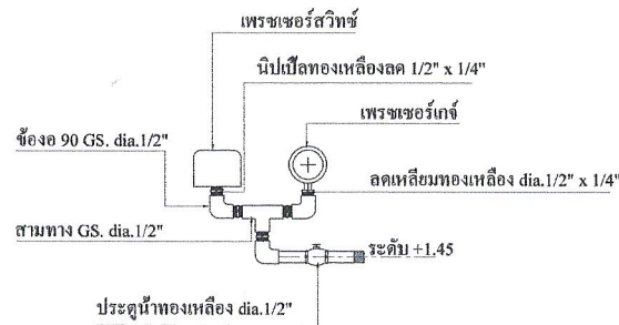
แบบขยายสวิทช์ควบคุมและเกย์วัดความดัน
