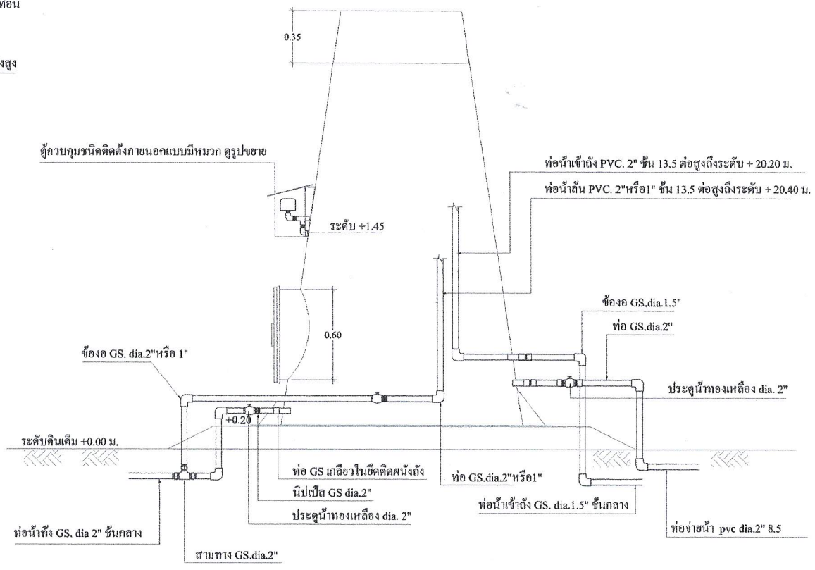
แบบแสดงการเดินท่อในถังแชมเปอญ มาตราส่วน 1 : 25
