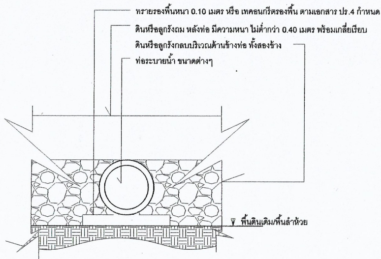
รูปตัดวางท่อระบายน้ำ NO SCALE
