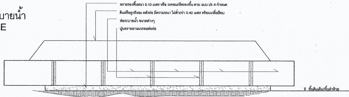
รูปตัดวางท่อระบายน้ำ NO SCALE
