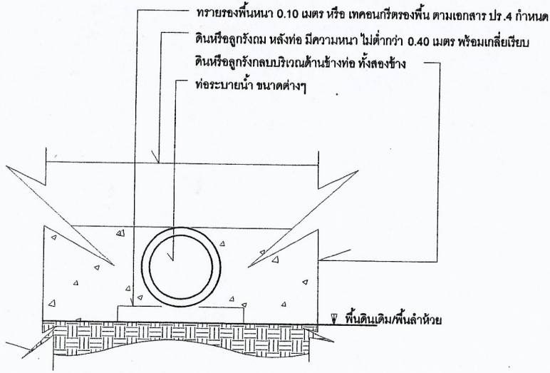
รูปตัดขวางท่อระบายน้ำ NO SCALE
